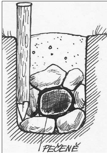
Tak zvaný Setonův hrnc se používá k vaření bez pomoci nádob. Kresba Jiří PETRÁČEK
